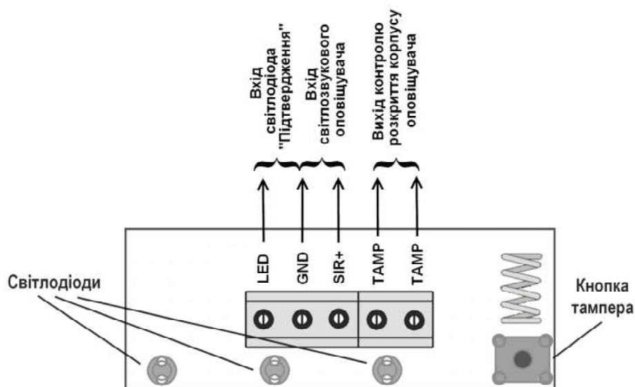
Рисунок 3 - Схема підключення оповіщувача
