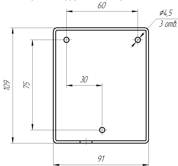
Рисунок 2 – Розмітка отворів на основі корпусу оповіщувача
