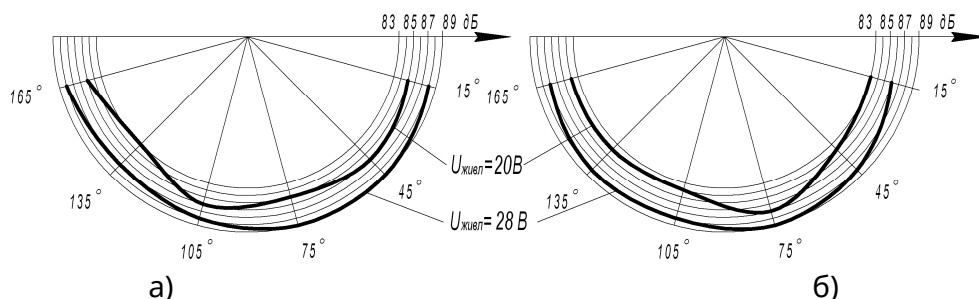
Рисунок 1 – Акустичні діаграми оповіщувача:
