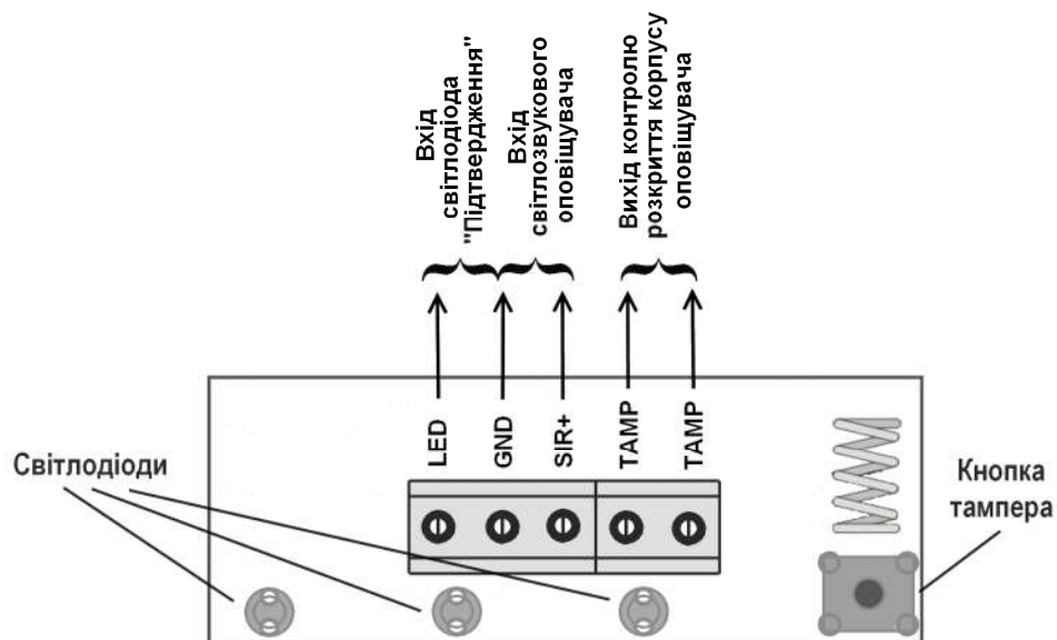
Рисунок 3 - Схема підключення оповіщувача
