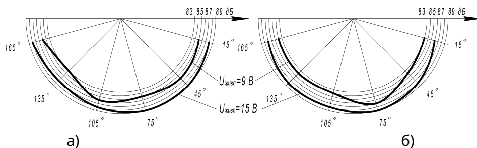
Рисунок 1 – Акустичні діаграми оповіщувача:
