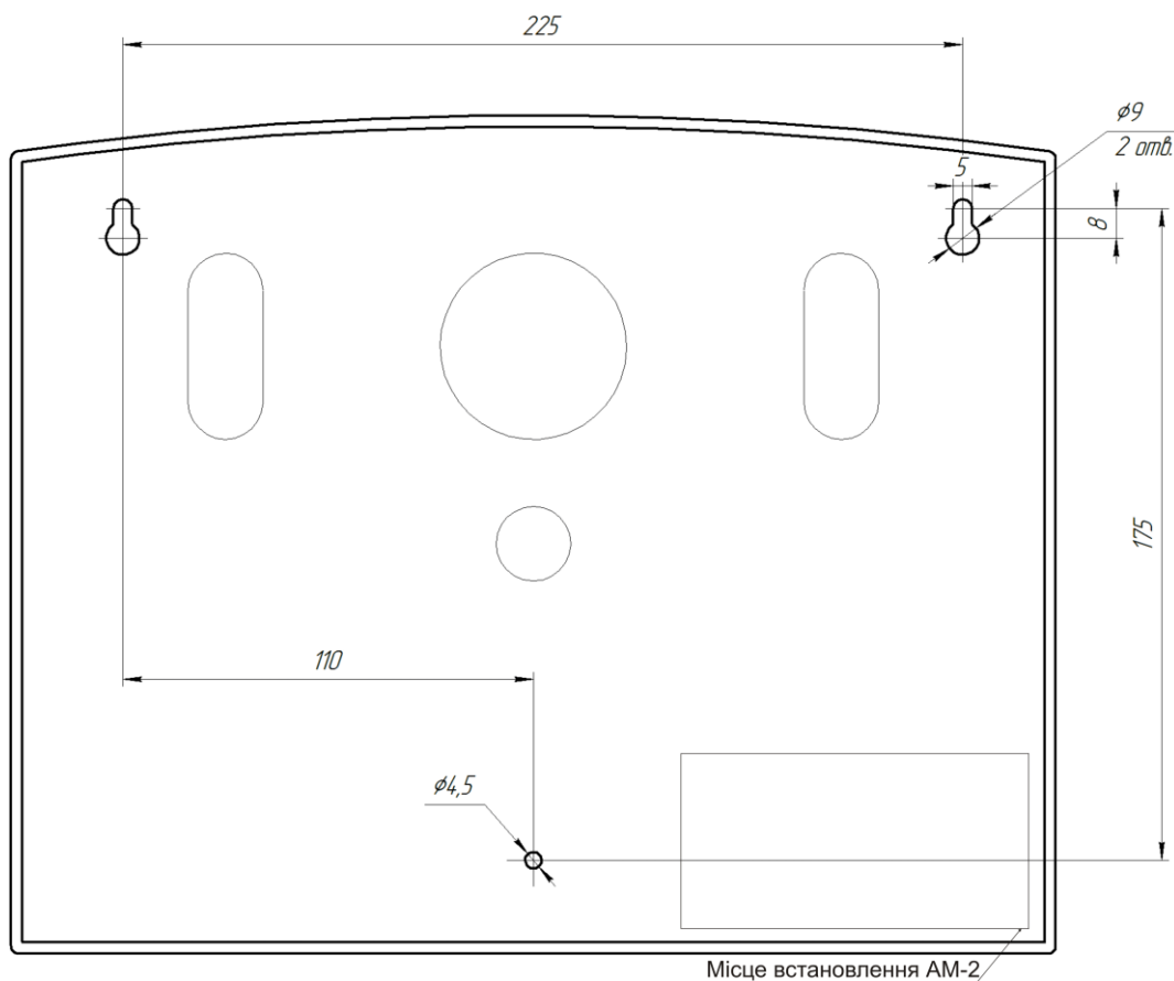
Рисунок 4 – Розмітка корпусу АПР
