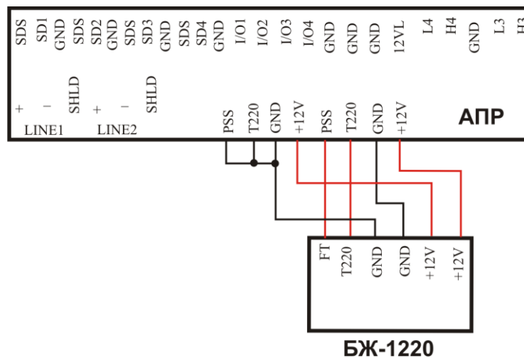
Рисунок 3 – Приклад підключення зовнішнього блоку живлення до АПР
