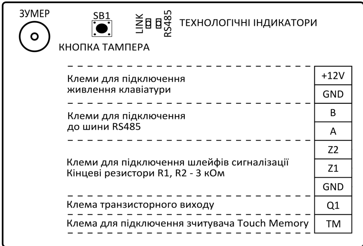
Рисунок 2 - Схема електрична підключення
