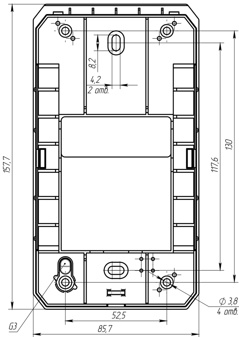
Рисунок 1 – Установчі розміри клавіатури
