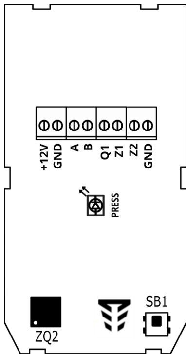
Рисунок 2 - Зовнішній вигляд та опис елементів плати клавіатури
