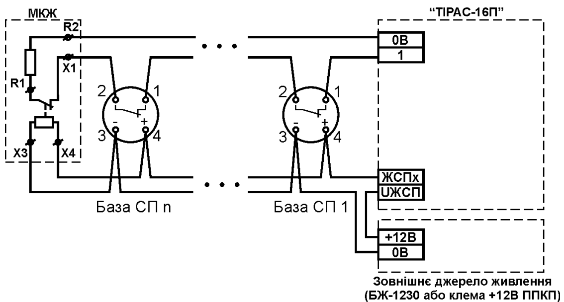
Рисунок А.4 – підключення живлення сповіщувачів
