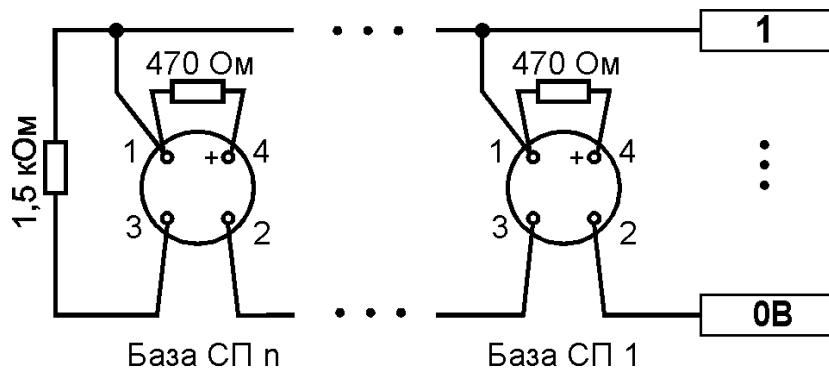
Рисунок А.3 – приклад підключення 2-х провідних сповіщувачів СП-4Т до 1 зони. Контакт «1» СП пустий, призначений тільки для кріплення додаткового резистора.
