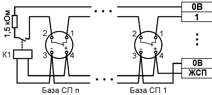
Рисунок А.2 – приклад підключення 4-х провідних сповіщувачів СП-1Т до 1 зони. К1 – реле з номінальною напругою 12В та нормально розімкнутим контактом). Шунтуючий резистор 2,2 кОм встановлюється між контактами 1 та 2 сповіщувача (не в базі).
