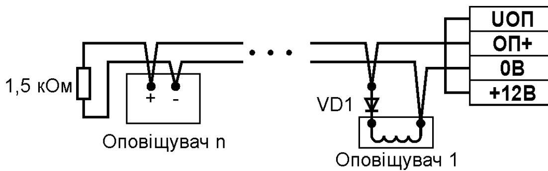
Рисунок А.5 – приклад живлення оповіщувачів від внутрішнього джерела живлення. Кінцевий резистор 1,5 кОм встановлюється в корпусі останнього в лінії оповіщувача.
