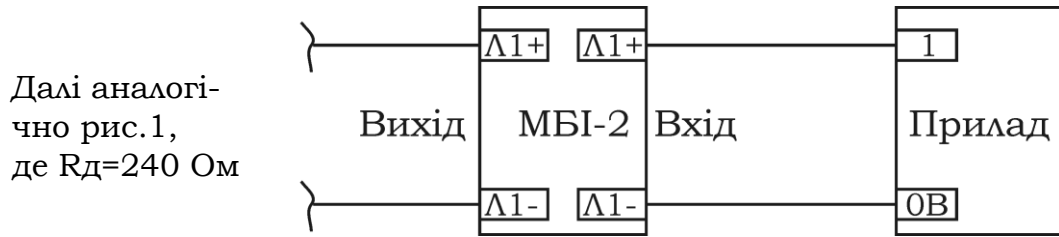
Рисунок А.5 – Схема підключення модуля МБІ-2 в першу зону приладу
