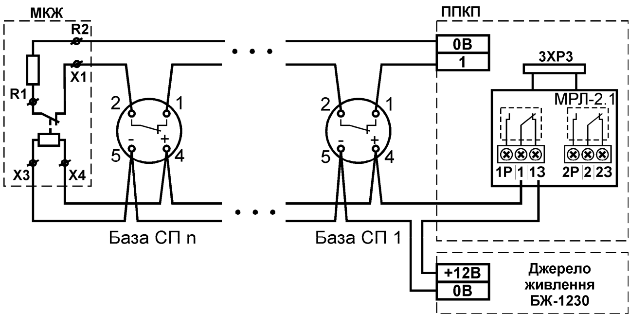
Рисунок А.9 – Схема підключення сповіщувачів СПД1-Тірас в першу зону ППКП через зовнішнє джерело живлення (в секції 02 повинні бути погашені всі зони, заводська настройка).
