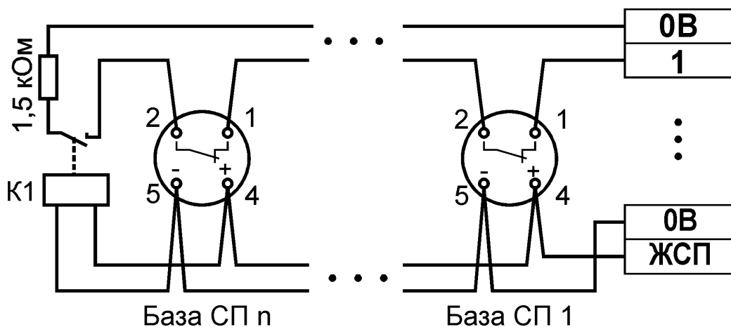
Рисунок А.5 – приклад підключення 4-х провідних сповіщувачів СПД1-Тірас до зони 1 від внутрішнього джерела живлення (К1 – реле з номінальною напругою 12В та нормально розімкнутим контактом). Шунтуючий резистор 2,2 кОм встановлюється між контактами 1 та 2 сповіщувача (на самому сповіщувачі, не в базі).
