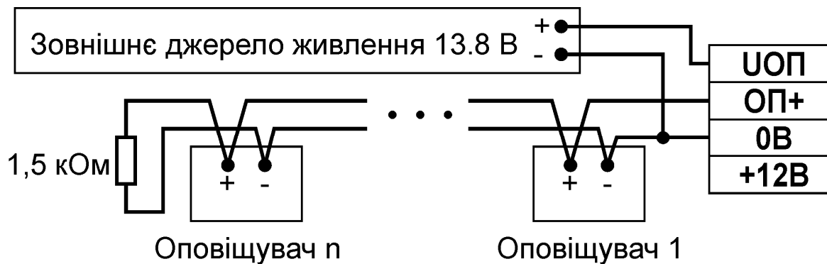
Рисунок А.4 – підключення оповіщувачів від зовнішнього джерела живлення (у випадку якщо струм навантажування виходу +12В при включенні оповіщення буде перевищувати 1 А).
