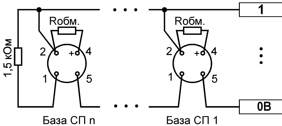
Рисунок А.6 – приклад підключення сповіщувачів СПД-2 Тирас до зони 1.
