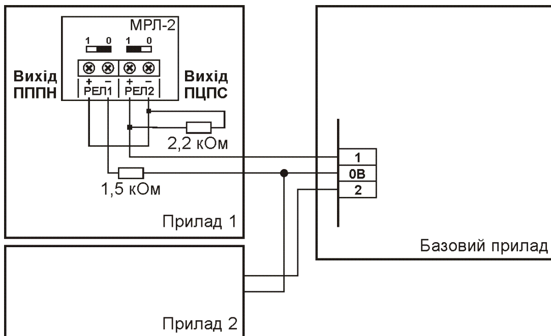
Рисунок А.7 – Підключення приладів „Тірас-ІІ” каскадом (наприклад для передачі сповіщень на пульт централізованого спостереження від декількох приладів по одній лінії зв’язку).
