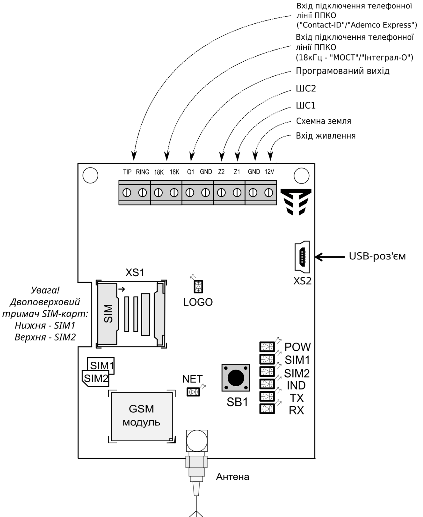
Рисунок А.1 – Схема підключення
