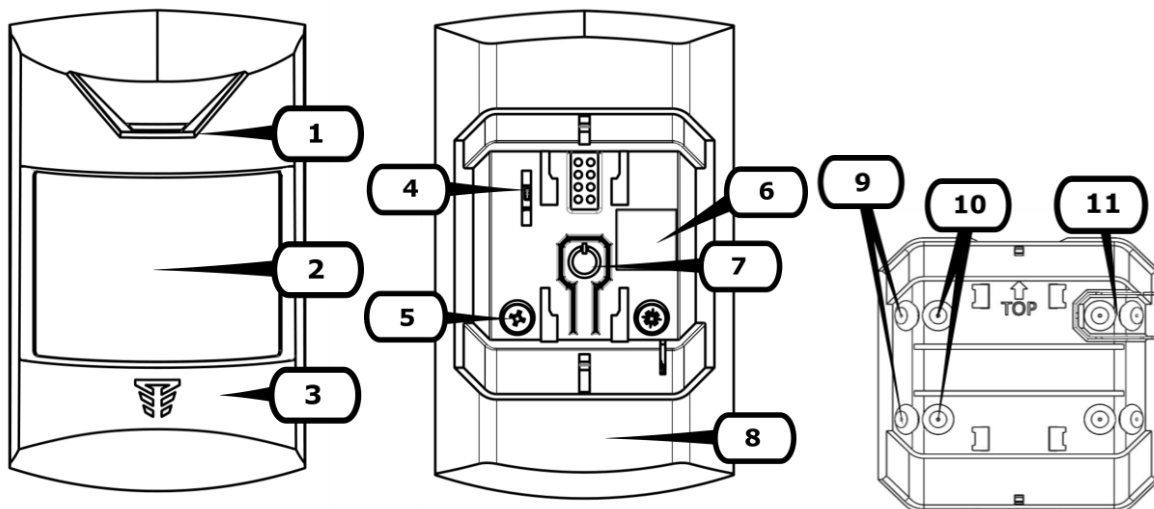
Рисунок 3 - Зовнішній вигляд елементів сповіщувача
