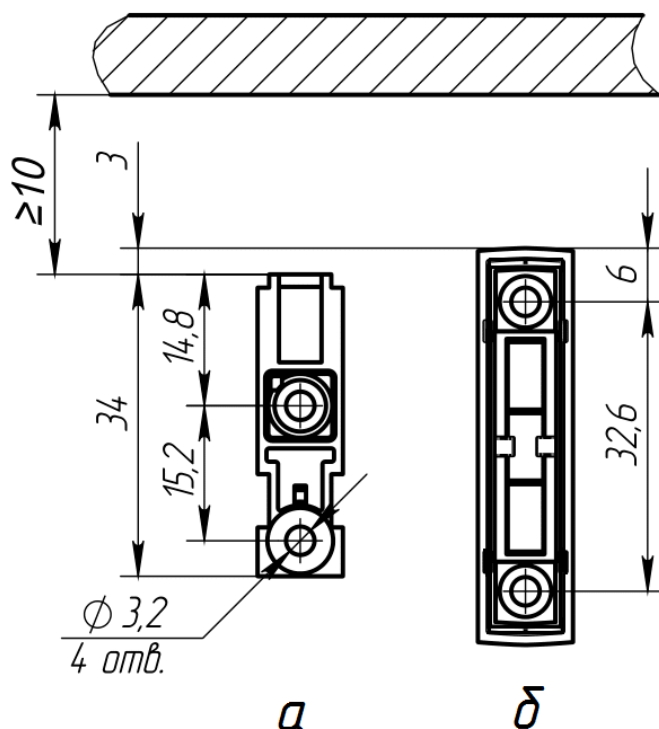
Рисунок 2 – Установчі розміри для сповіщувача та магніта
